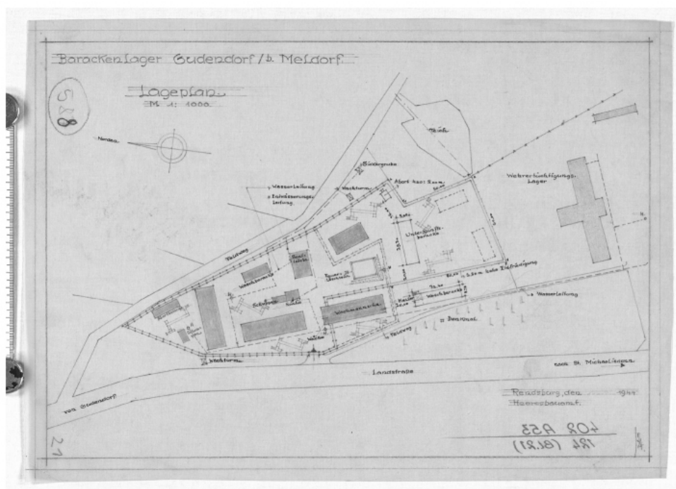
Plan sytuacyjny obozu z barakami w Gudendorf k. Meldorf, wykonany przez Urząd Budowlany Wojsk Lądowych w Rendsburgu w 1944 r. Źródło: Schleswig-Holsteinisches Landesarchiv, Abt. 402, A 53, Nr. 124, Blatt 21
